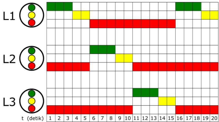
Gambar II.10. Skema diagram waktu lampu rambu lalu-lintas 1.
